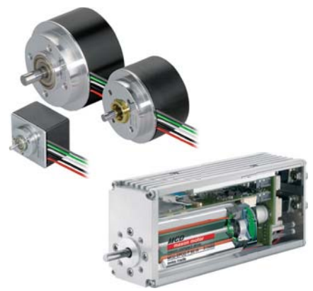
maxon motor Kompaktssysteme
