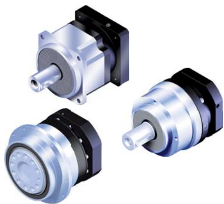
Apex Getriebe der AB, AD und AE Reihe
